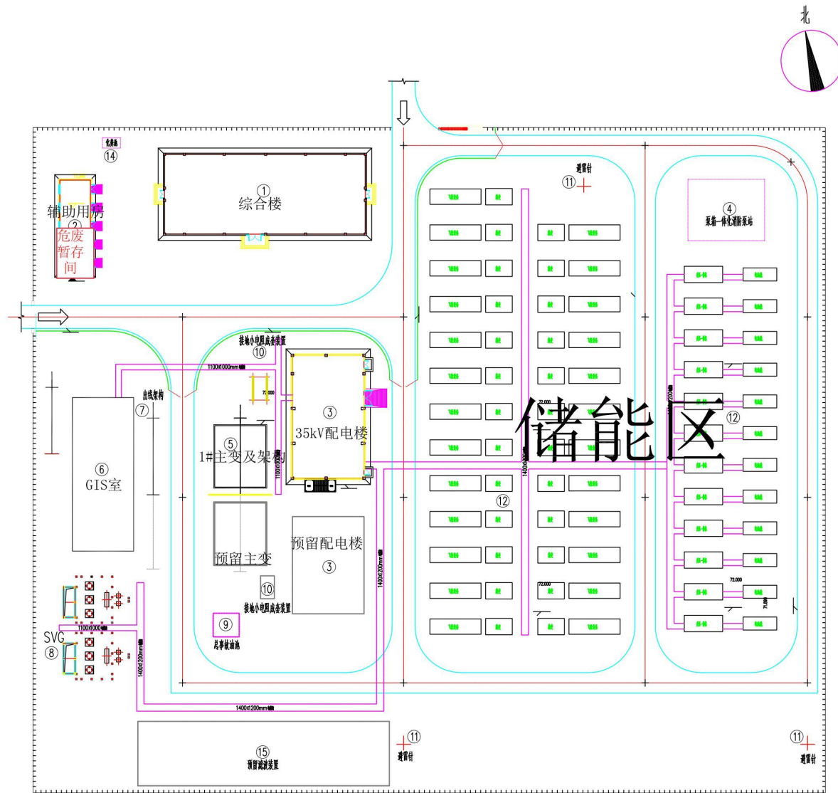
附图3 本项目升压站总平面布置图
