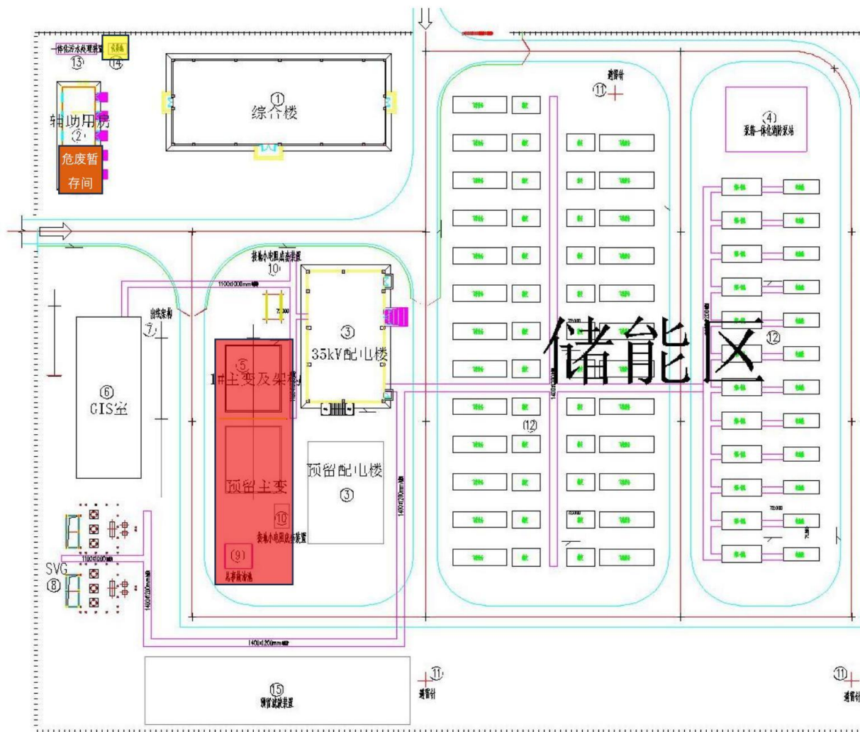
附图7 本项目升压站分区防渗示意图
