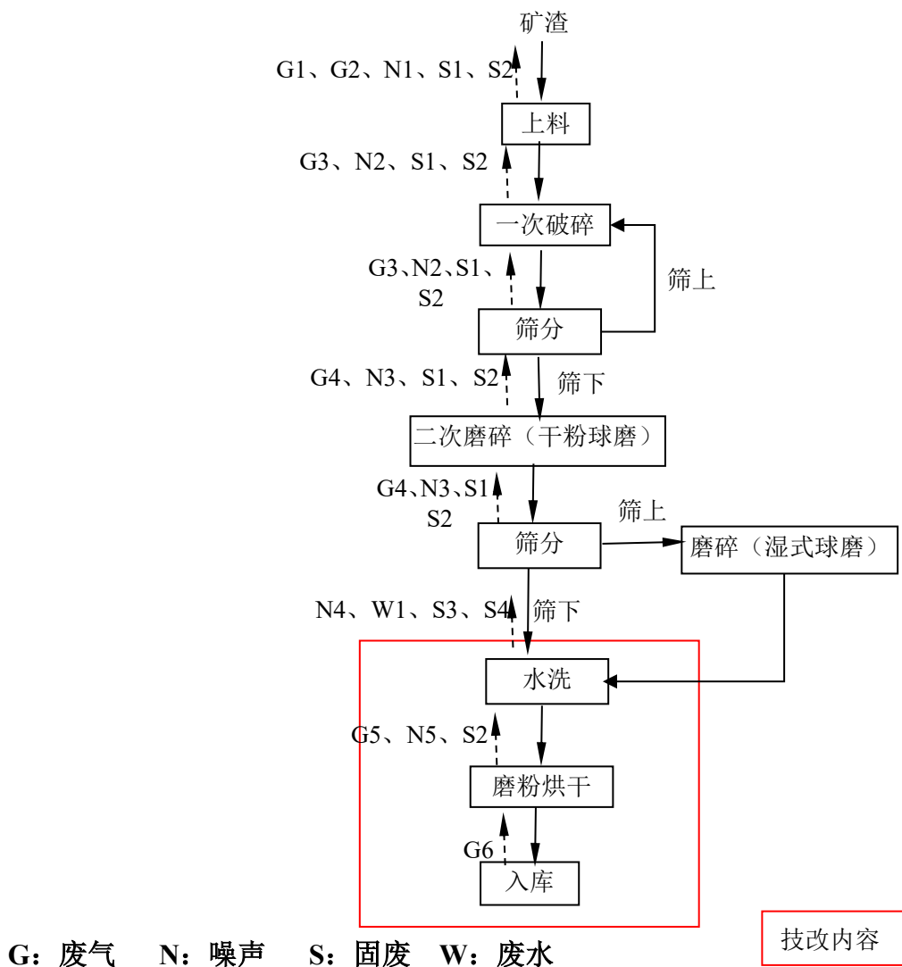
图 2-2 本项目生产工艺流程及排污节点图
