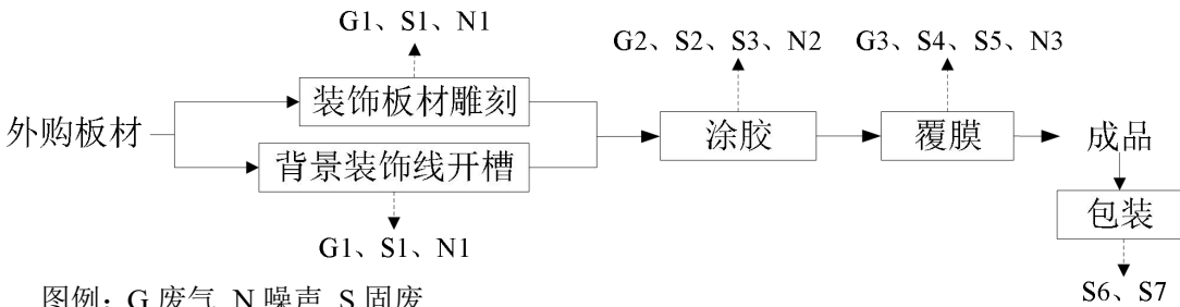
图 3 项目新型环保装饰板材、背景装饰线生产工艺流程及排污节点图
