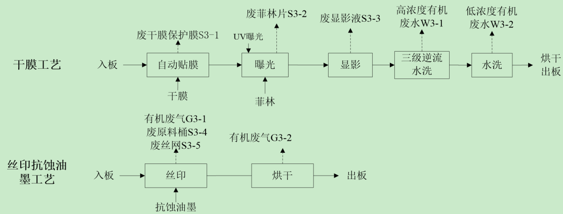
图 2-7 图形制作工艺流程
