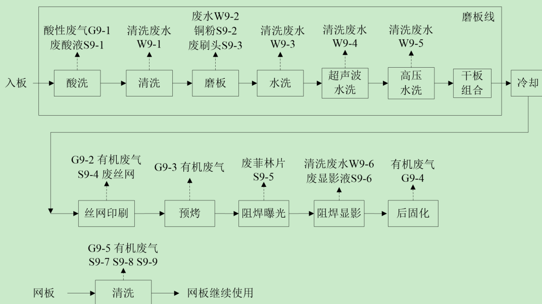
图 2-13 阻焊工艺流程
